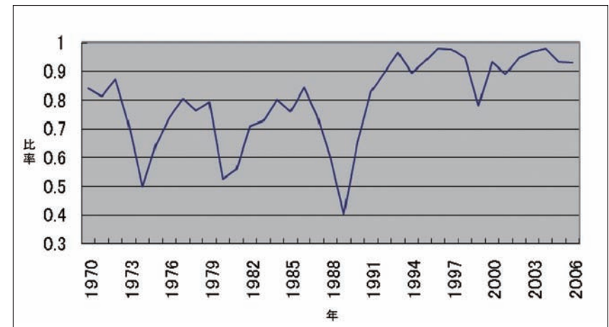
図9 マサバ太平洋系群漁獲物の年齢構成（データ：川端ら 2012）
