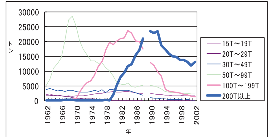
図8 北まき付属船の階層別総トン数の推移（データ：漁船統計）
