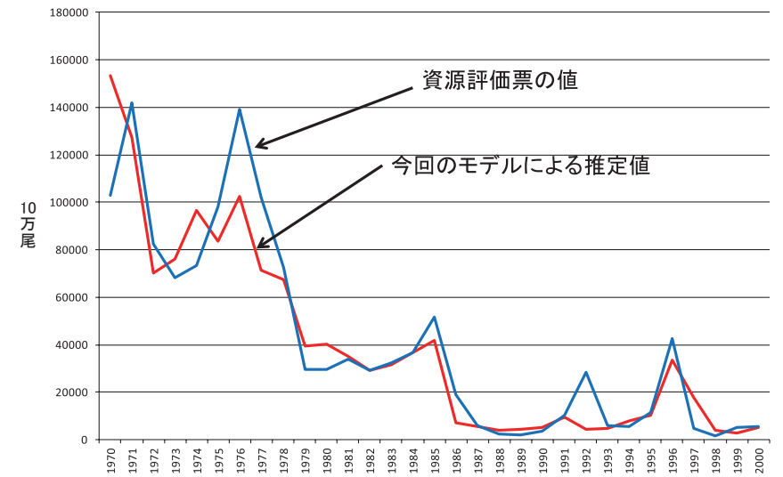
図13 Extended Ricker Model を用いたマサバ太平洋系群加入尾数の推定結果 (牧野・金子 2013 を基に作成)
