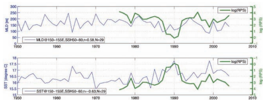
図4 混合層深度(上)および海面水温(下)とマイワシ再生産(log(RPS))の関係(Nishikawa et al. 2011 を一部改編)
