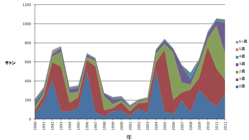
図12 マサバ太平洋系群資源量の推移（データ：川端ら 2012）
